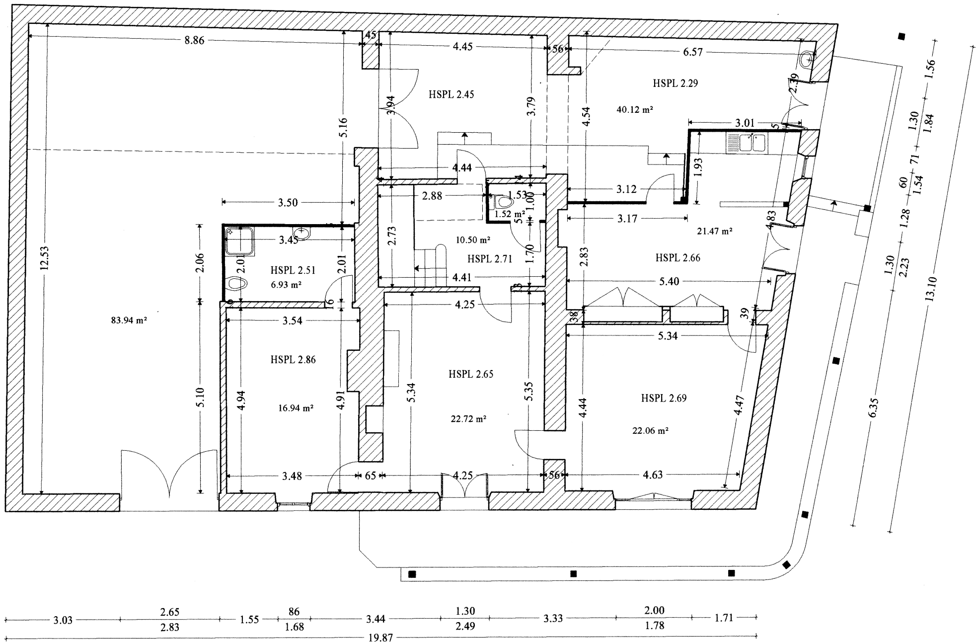
PLAN REZ DE CHAUSSEE EXISTANT ECHELLE 1/100
